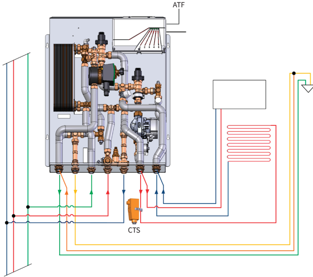
Fig. : Exemple d'intégration d'une station LogoMatic G2 MC-UC-DHWC avec circuit de chauffage mélangé ainsi que CTS et STE en option.
