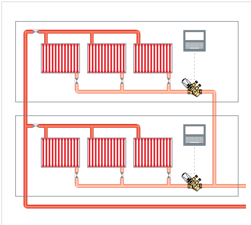
Exemple d'application 3 - Installation de chauffage central
